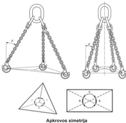
Apkrovos simetrija
