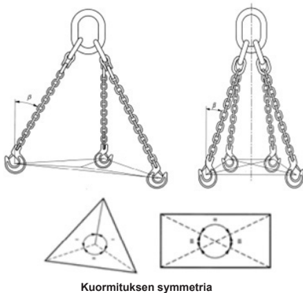
Kuormituksen symmetria
