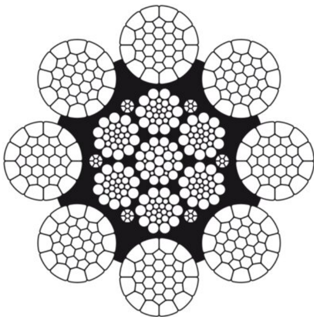
Bovenloop-kraan
